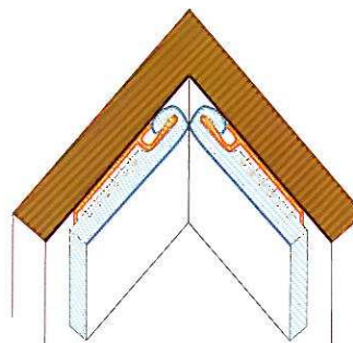
2 angle rentrant
